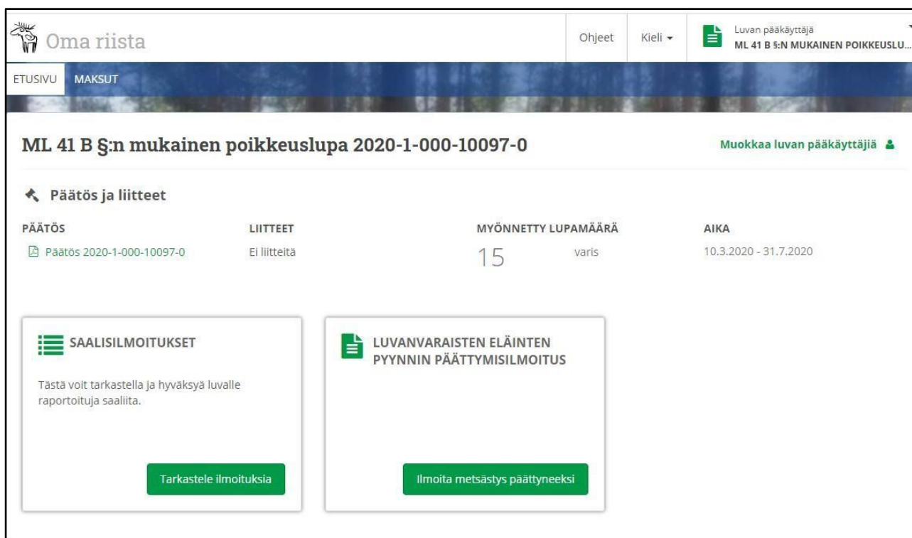
Kuva 4. Luvan pääkäyttäjänäkymä
