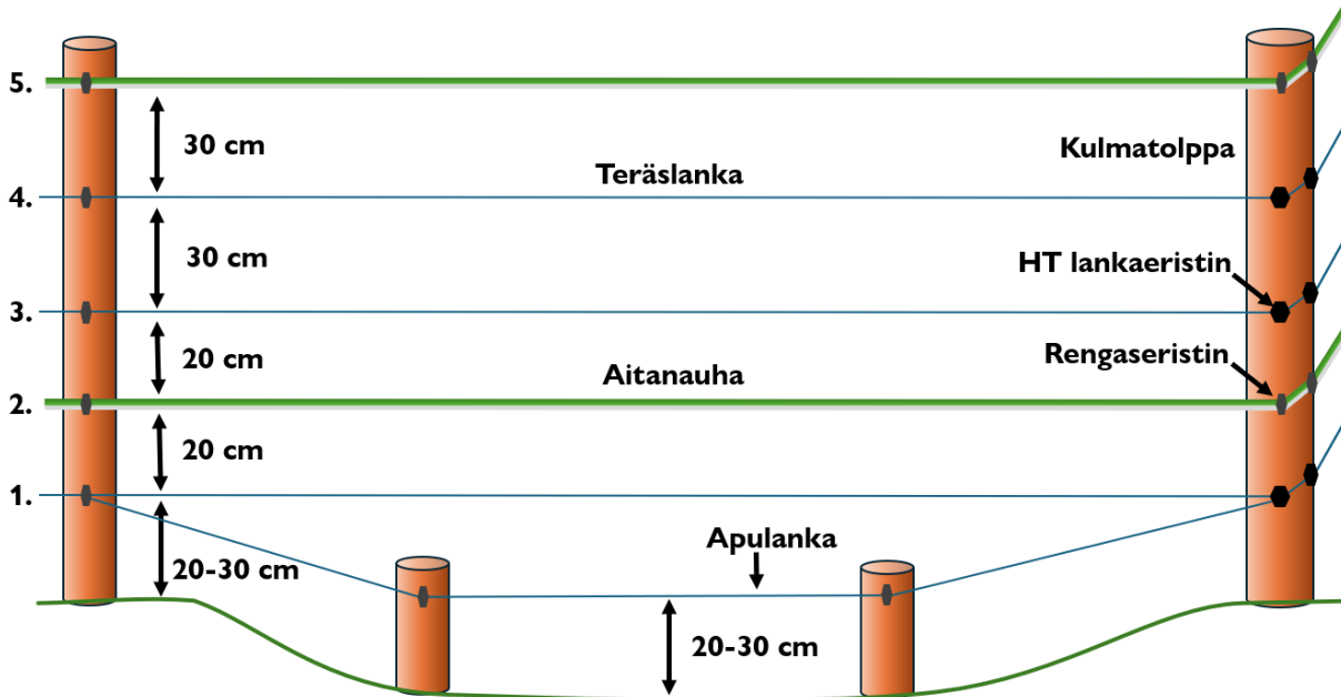
Kuva 1. Petoaidan rakennepiirros ja apulangan asentaminen painanteen kohdalla.
